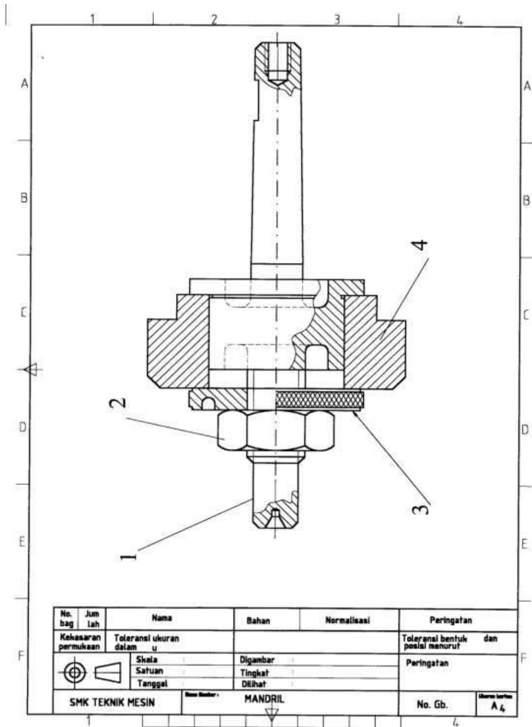
Gambar 6.7(Mandril)
