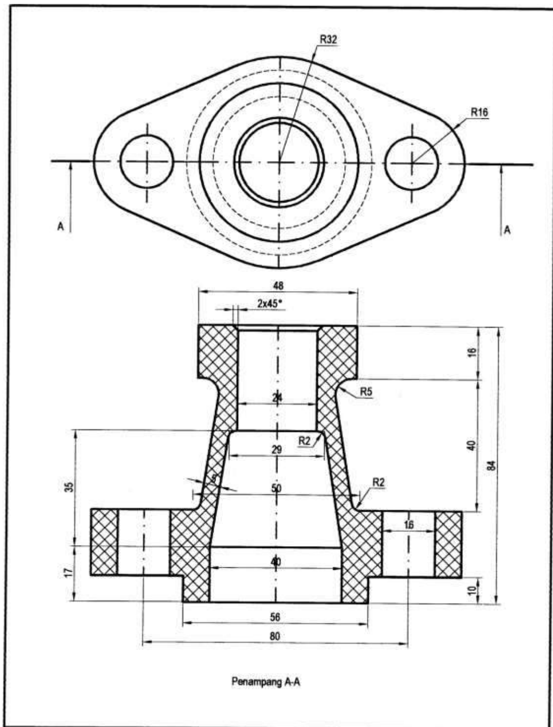
Gambar 5.7 /dudukan katup
