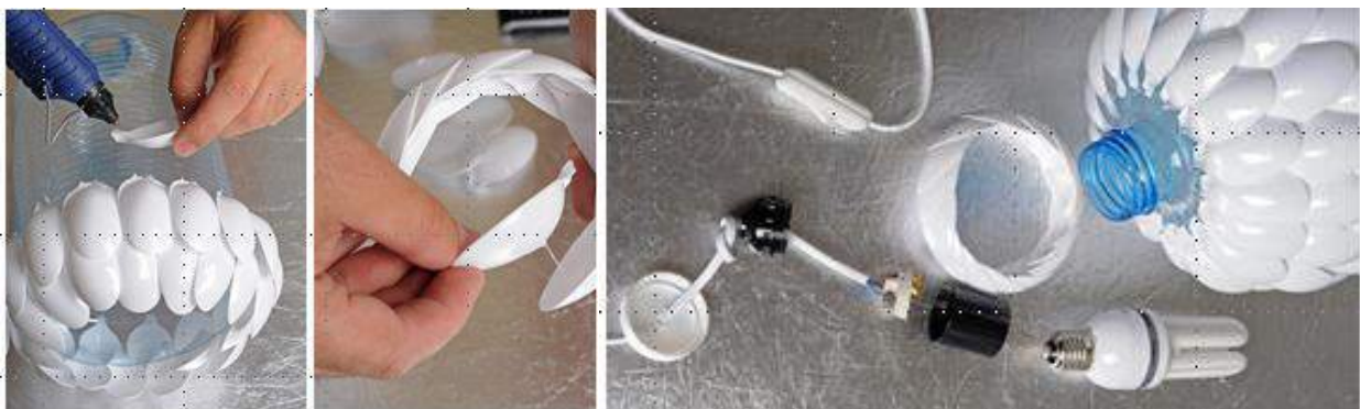
Gambar 4. Proses pembuatan lampu meja kerja Sumber: penulis, 2020
