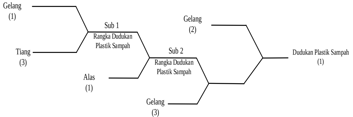
Gambar 13. Diagram Perakitan Rangka Estetis Dudukan Plastik Kantong Sampah Berbahan Besi Nako
