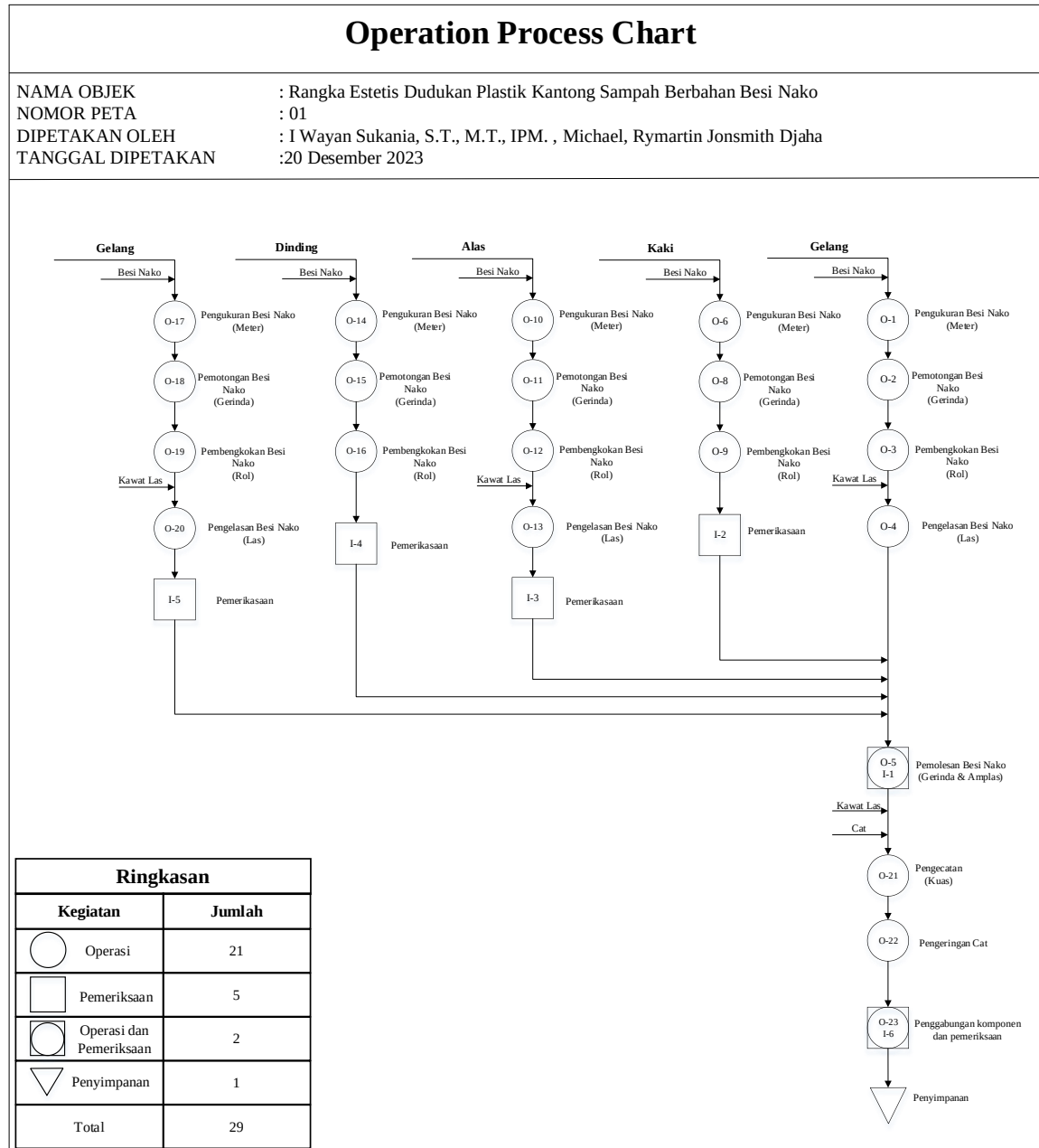
Gambar 18. OPC Rangka Estetis Dudukan Plastik Kantong Sampah Berbahan Besi Nako
