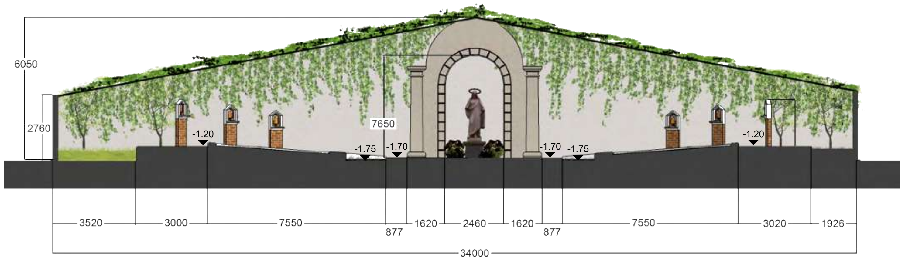
POTONGAN B-B' AREA DOA MARIA ALT 1
