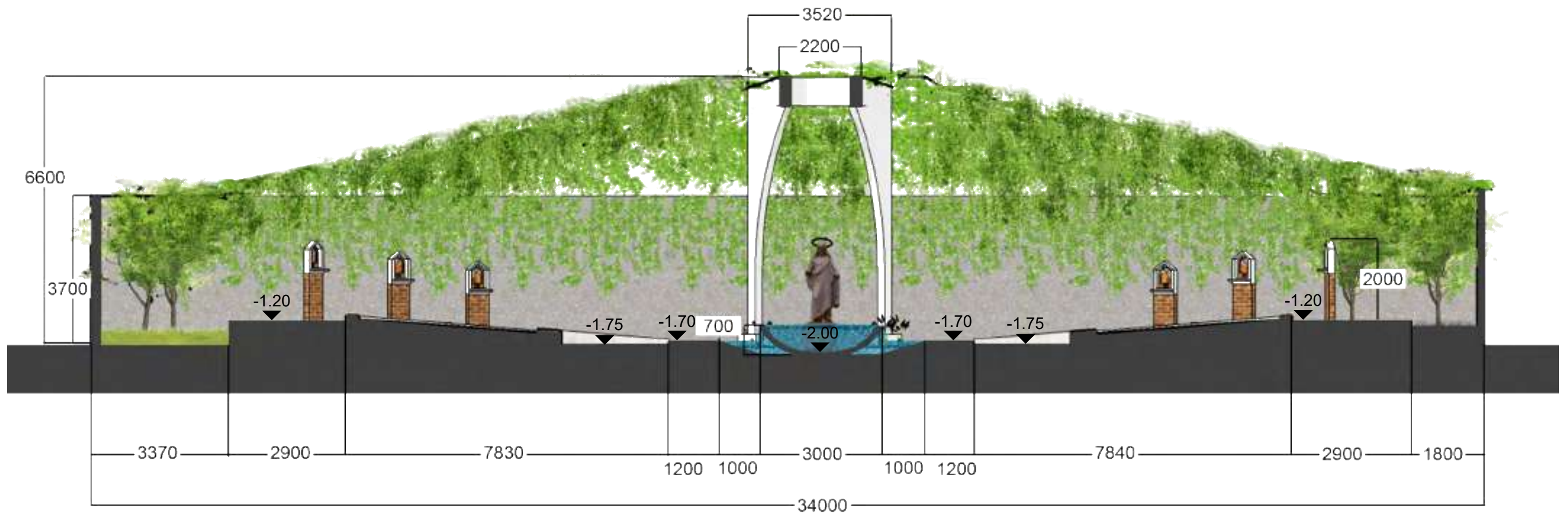
POTONGAN B-B' AREA DOA MARIA ALT 3
