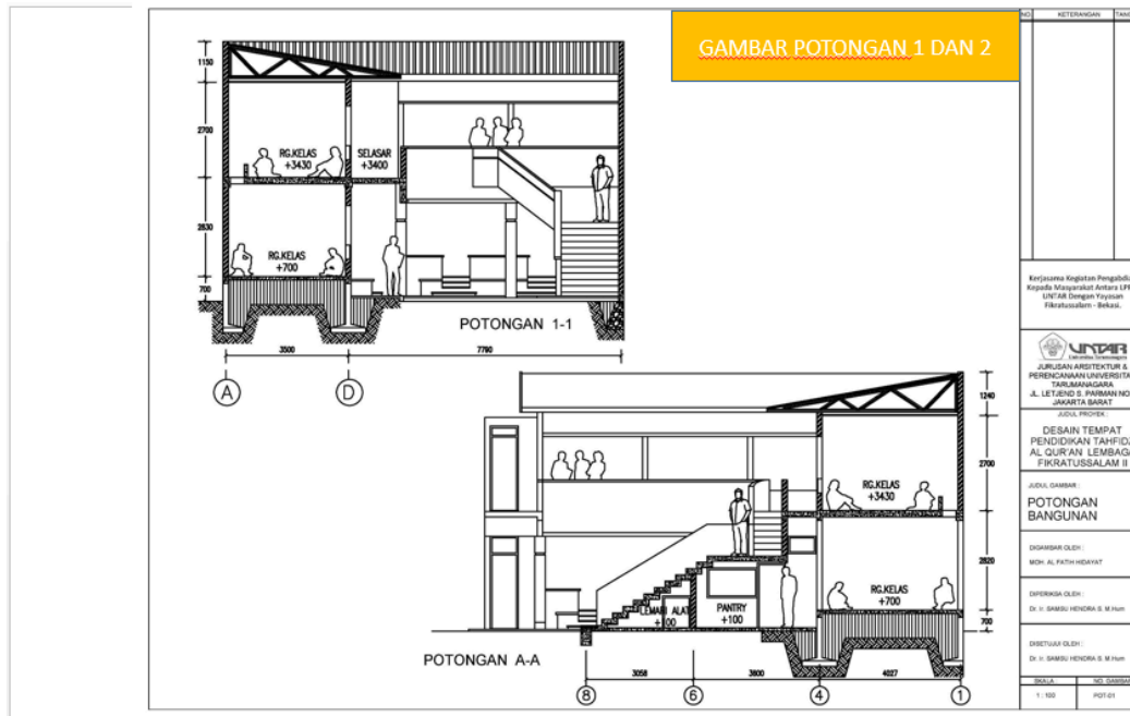
Gambar 8. Potongan Bangunan Fiktarusalam II
