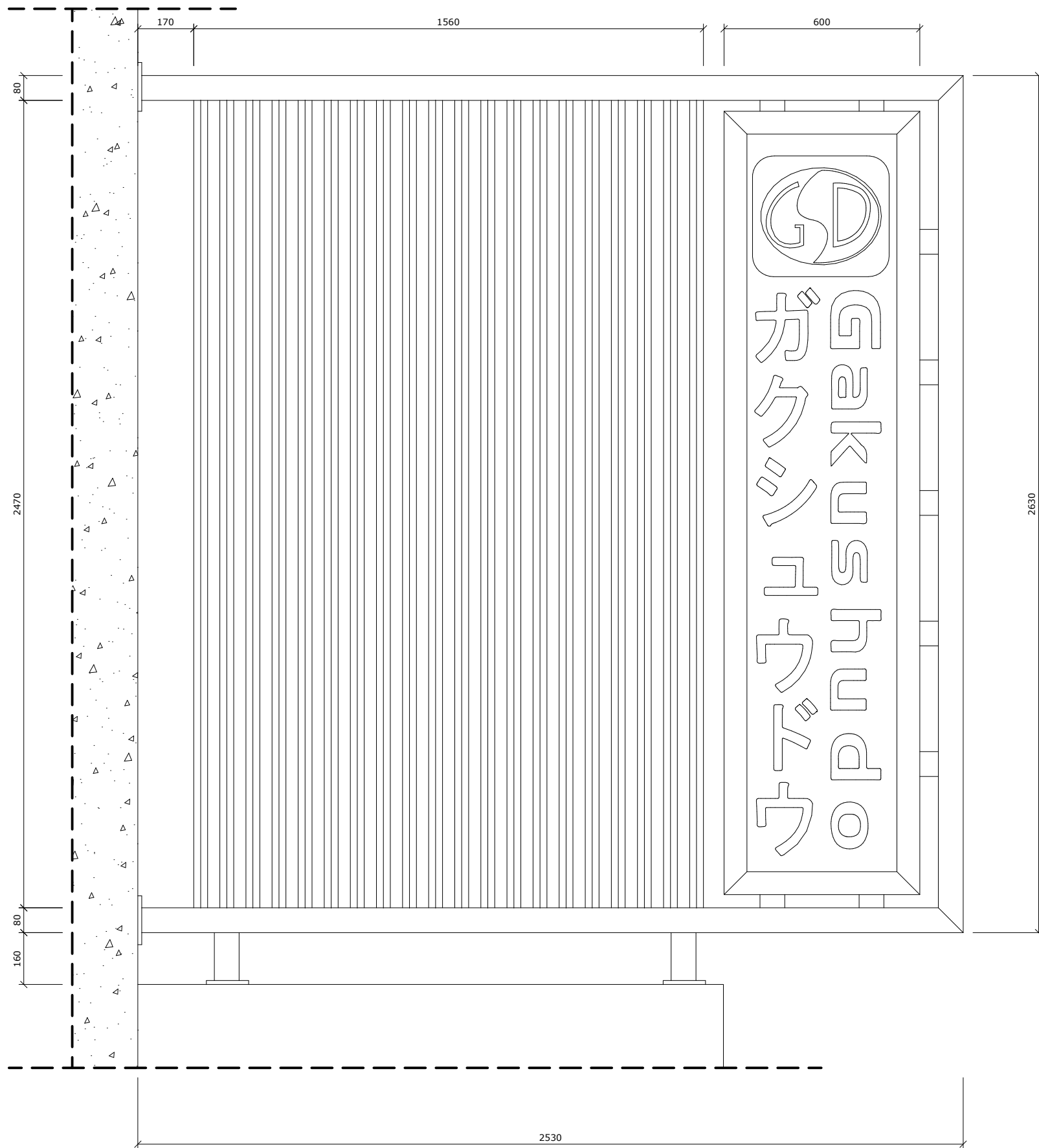
A 1 TAMPAK DEPAN 1:15
