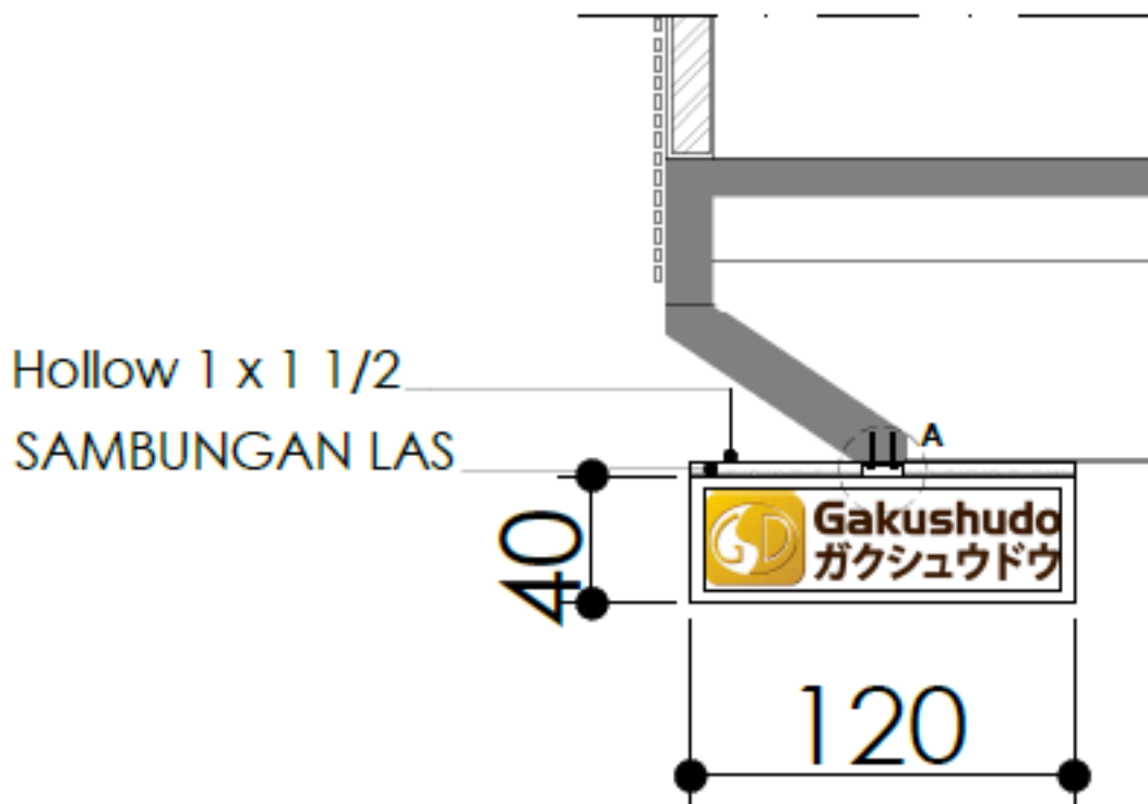
Gambar 2. Posisi pemasangan Papan Reklame Bangunan Kantor Gakushudo.
