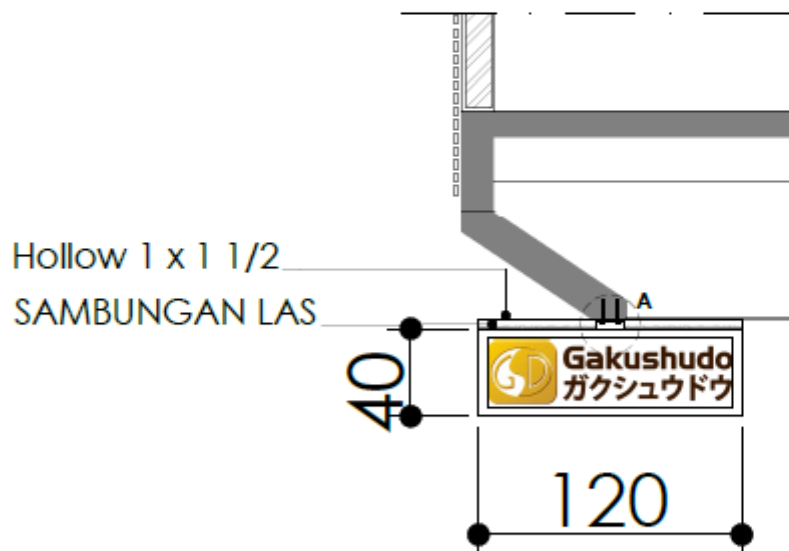
DETAIL PEMASANGAN REKLAME SKALA 1:25
