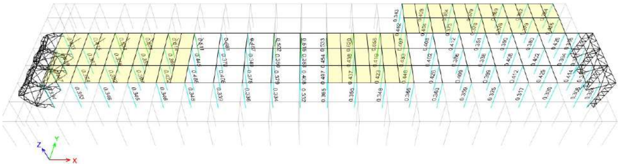
Gambar 4.6. Rasio Aksial-Lentur Kolom Lantai Atap
