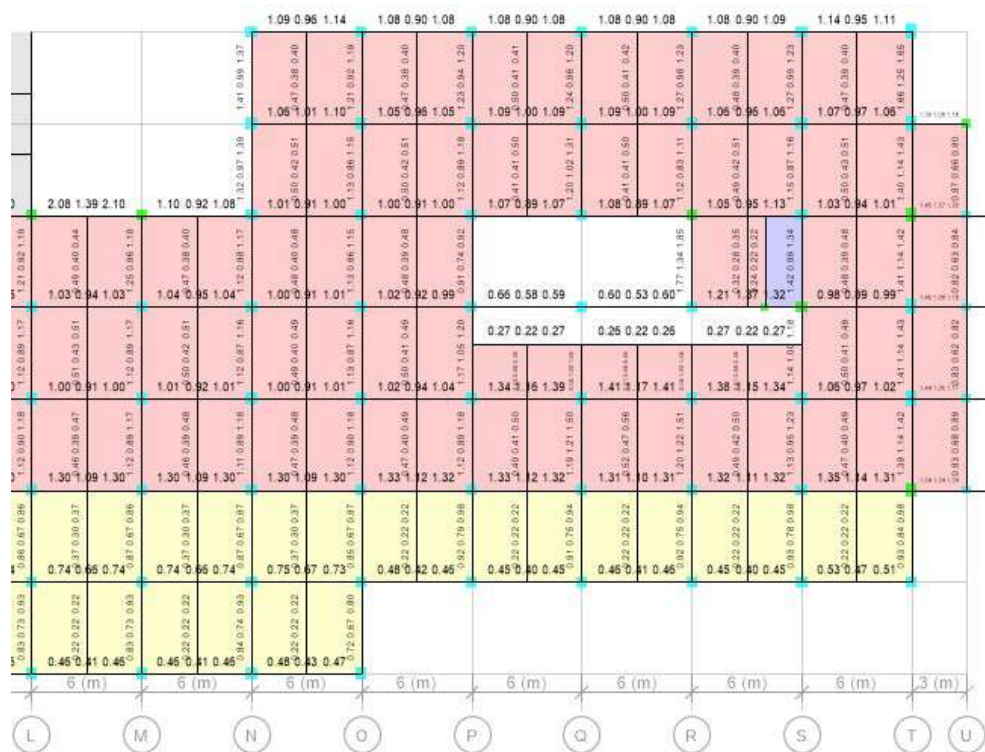
Gambar 4.13. Tulangan Geser Balok Lantai Dua
