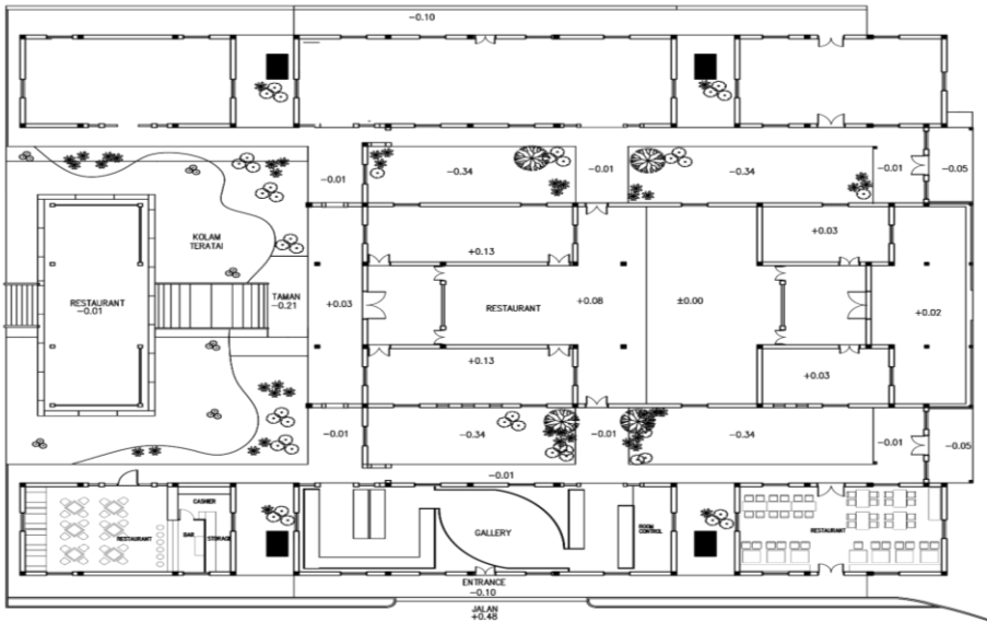
Gambar 3. Denah Bangunan Utama Candra Naya Sumber: Dokumentasi pribadi 2022
