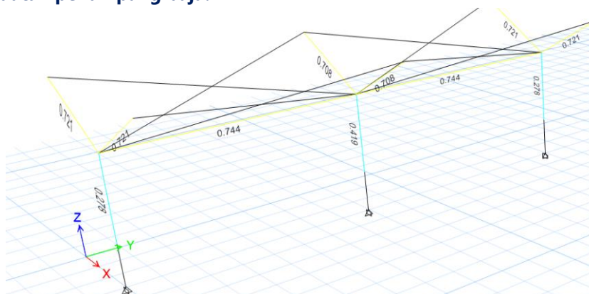
Rasio Kekuatan Baja, Nilai < 1.00 menunjukkan penampang mampu menahan gaya dalam yang terjadi
