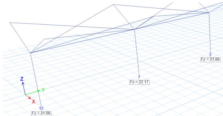
Reaksi kolom akibat kombinasi beban tetap, satuan kN
