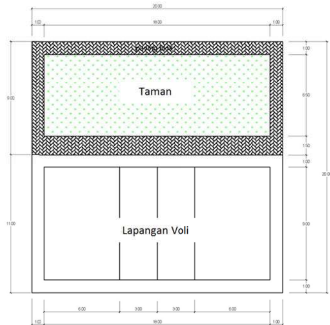
Gambar 2.5 Gambaran Awal Desain Fasilitas Olahraga dan Bermain Berdasarkan hasil Diskusi dengan Mitra (Sumber: Penulis, Juli 2022)
