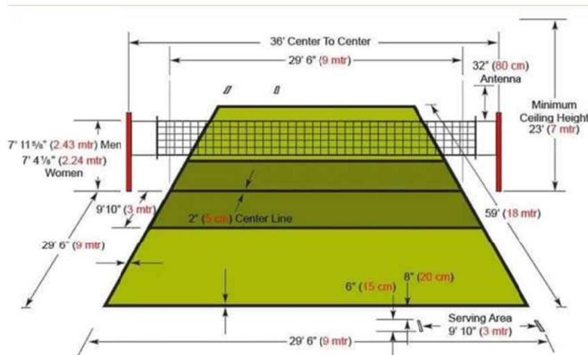
Gambar 2.1 Ukuran Lapangan Voli (Sumber: https://pastiguna.com/ukuran-lapangan-bola-voli/ )
