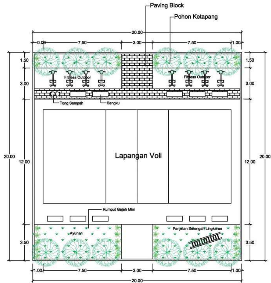
Gambar 4. Site Plan : (a) Alternatif 1 dan (b ) Alternatif 2 (Sumber: Desain Penulis, September 2022)
