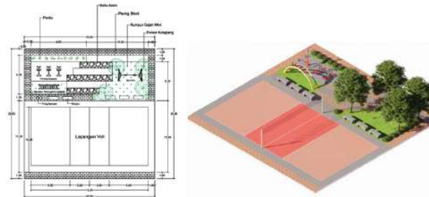
Gambar 2. Desain Fasum Blok B Perumahan BIP
