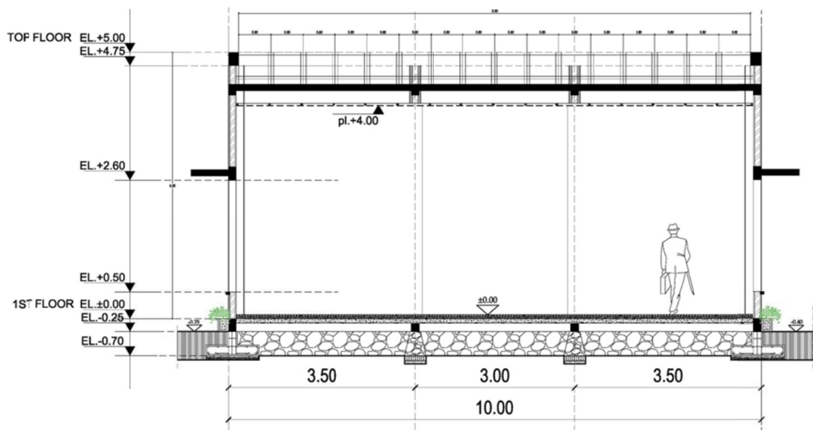
Gambar 2.2 Potongan A-A Mushola Al-Abror ( Scale to Fit ) (Sumber: Dokumentasi Mitra, Januari 2021)
