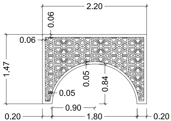
1 TAMPAK DEPAN SCALE 1:50
