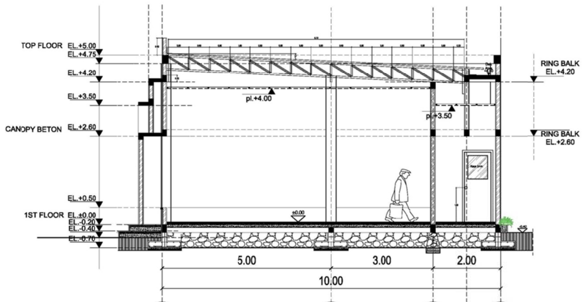
Gambar 2.3 Potongan B-B Mushola Al-Abror ( Scale to Fit ) (Sumber: Dokumentasi Mitra, Januari 2021)
