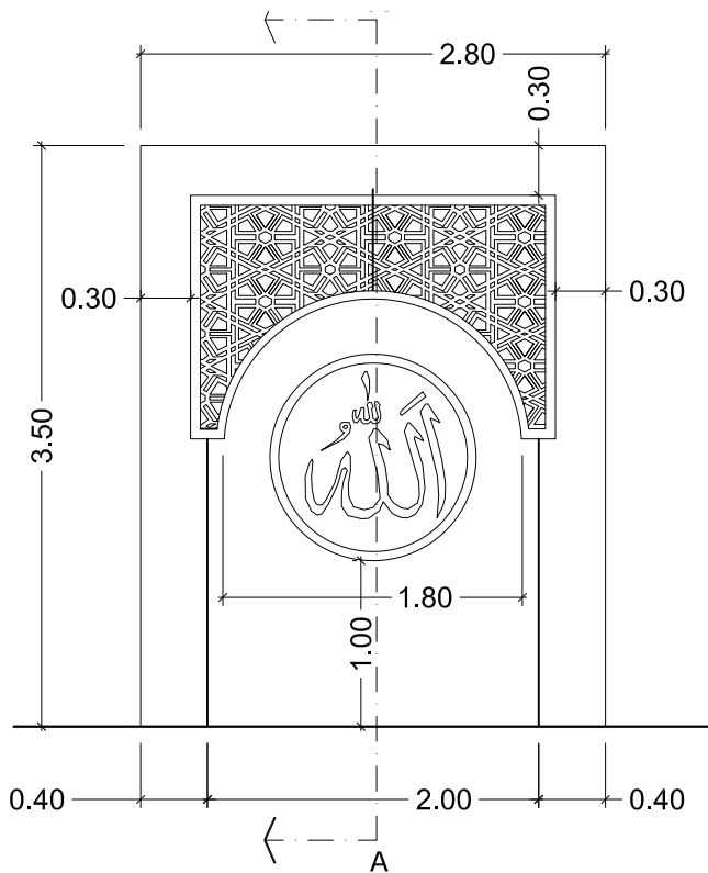
1 TAMPAK DEPAN SCALE 1:50
