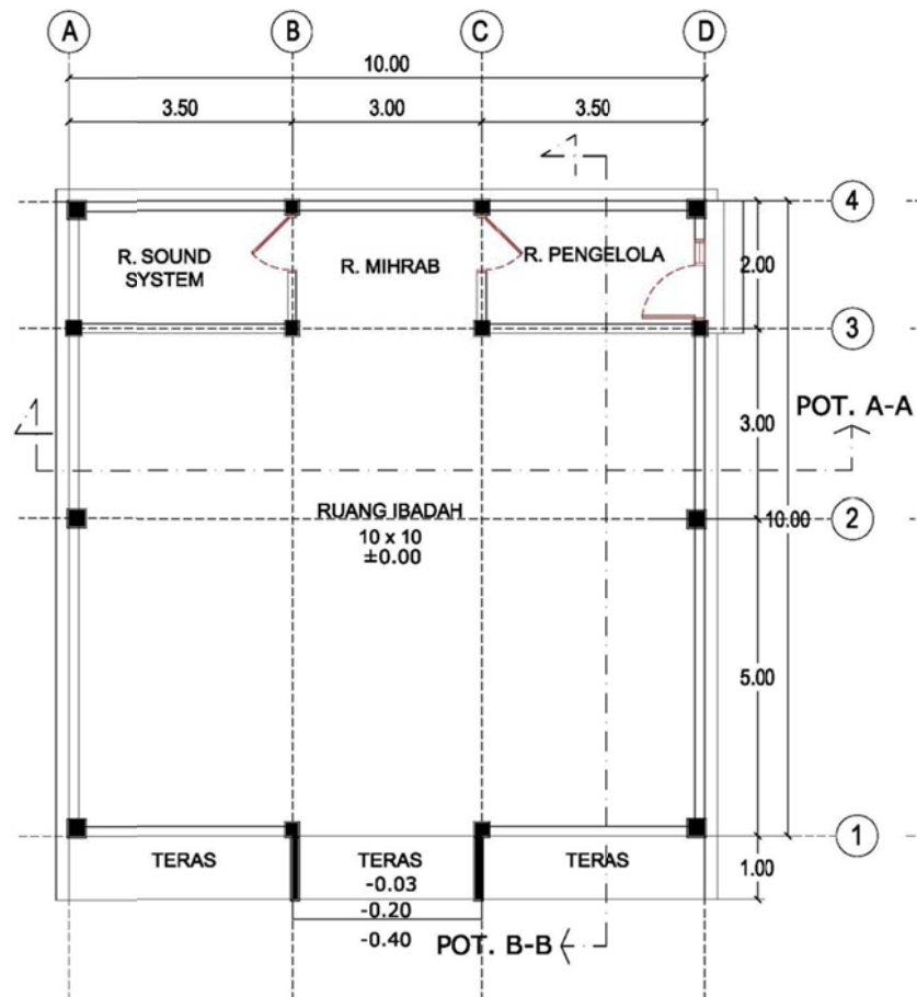
Gambar 2.1 Denah Mushola Al-Abror ( Scale to Fit ) (Sumber: Dokumentasi Mitra, Januari 2021)
