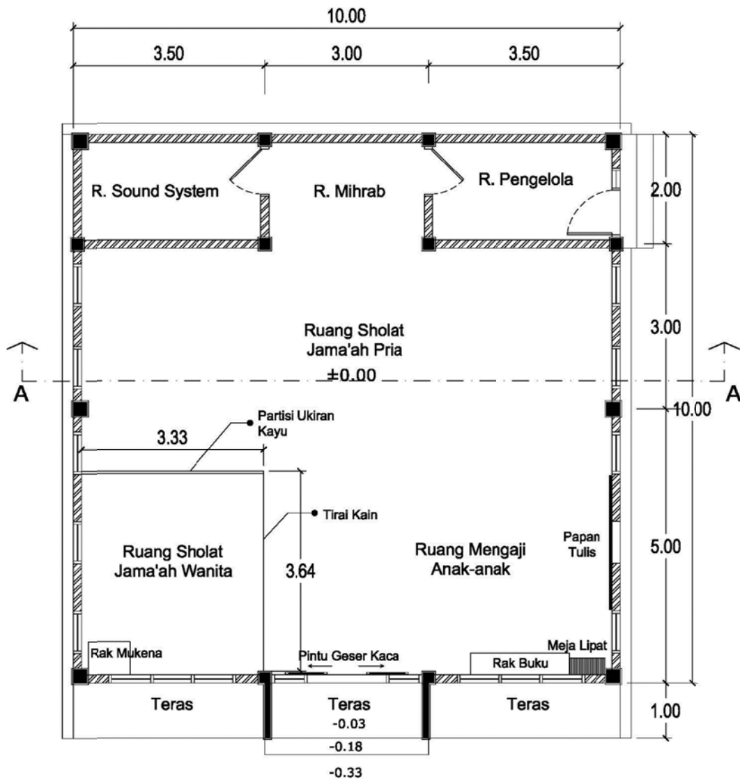
Gambar 4.1 Desain Denah Mushola Al-Abror ( Scale to Fit ) (Sumber: Penulis, Maret 2021)
