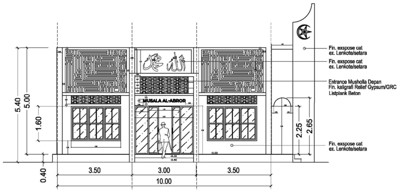
Gambar 1.13 Tampak Depan Mushola Al-Abror ( Scale to Fit ) (Sumber: Dokumentasi Mitra, Januari 2021)
