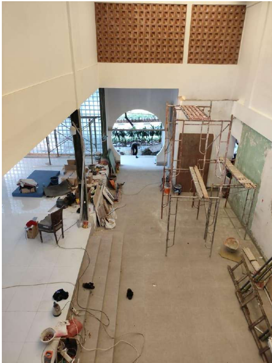
Gambar 13. Proses Pekerjaan Lantai Penghubung Bangunan Masjid dengan SMA Negeri di Lantai 1 sampai Minggu Pertama Agustus 2024
