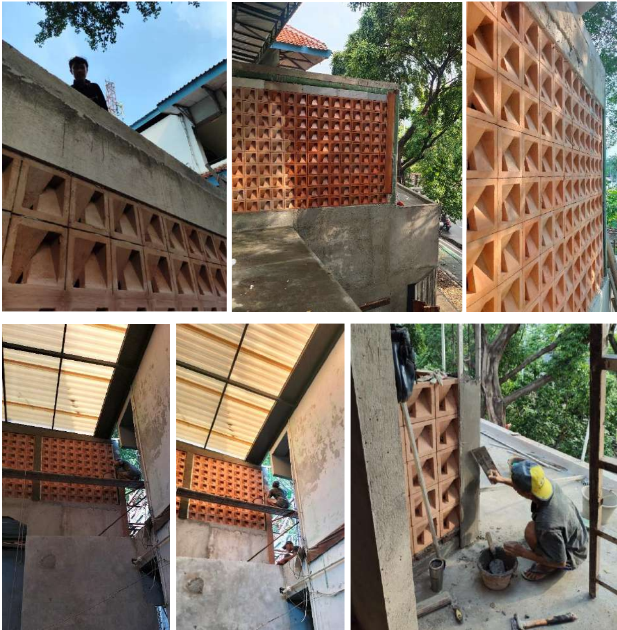
Gambar 8. Proses Pekerjaan Dinding Roster pada Lantai 2 sampai Minggu Kedua Juli 2024
