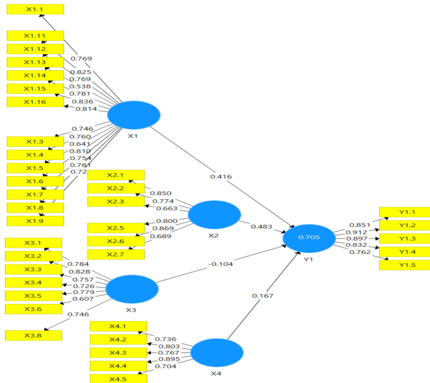
Gambar 3. Perhitungan lanjutan
