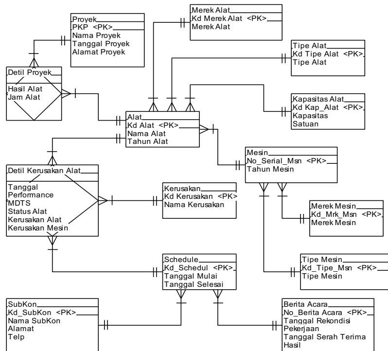
Gambar 2. Diagram Hubungan Antar Entitas.
