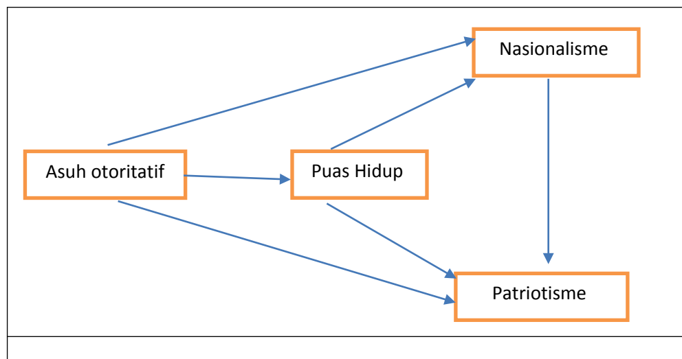
Gambar 1 Desain Penelitian
