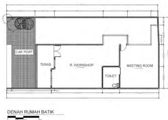
Denah Eksisting Rumah Batik Palbatu
