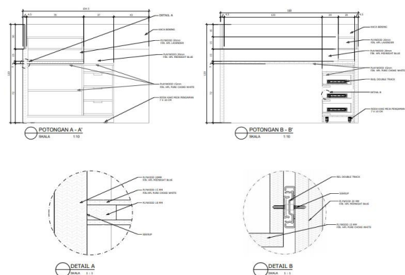
Gambar 9 : Potongan dan Detail
