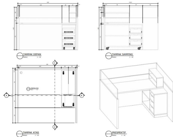
Gambar 8 : orthogonal dan isometri
