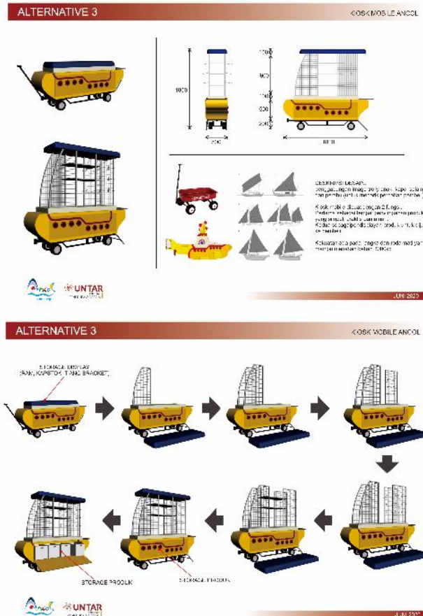
Gambar 6. (a) Desain kiosk mobile alternatif 3 dan (b) proses buka tutup display. Sumber: Penulis, 2020
