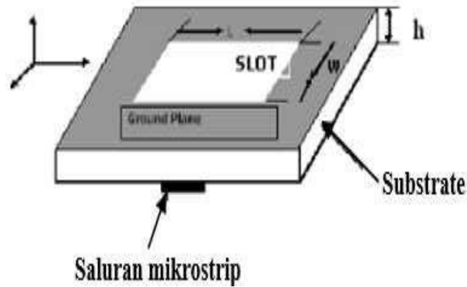
■ Gambar 2. Slot Antena Mikrostrip
