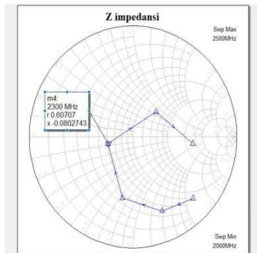
■ Gambar 10. Nilai Input Impedance
