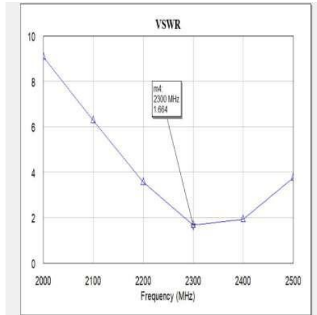
■ Gambar 9. Nilai VSWR
