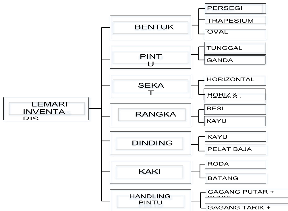
Gambar 3. Pohon Klasifikasi Konsep Lemari Inventaris Sumber: Sukania et al. (2020)
