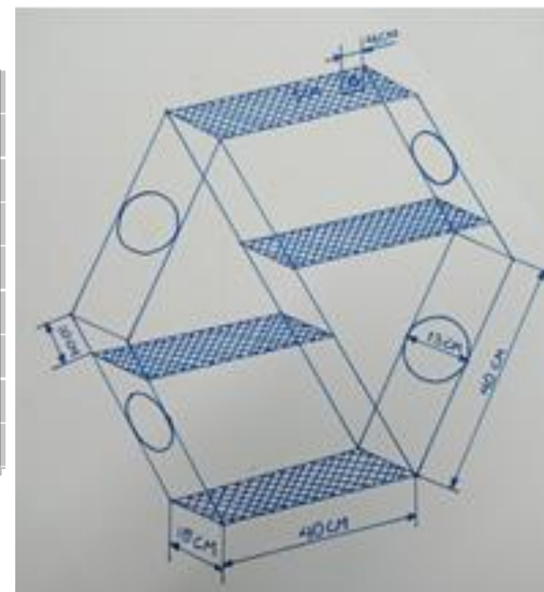
Gambar 3. Desain Rak Tempel Dinding Minimalis
