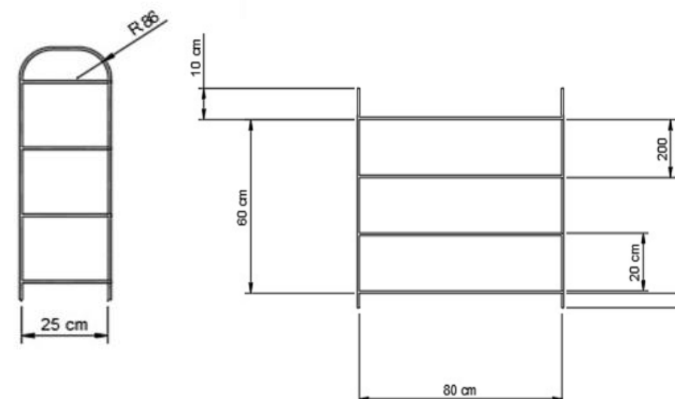
Gambar 1. Tahapan Perakitan Rak Sandal Model 1
