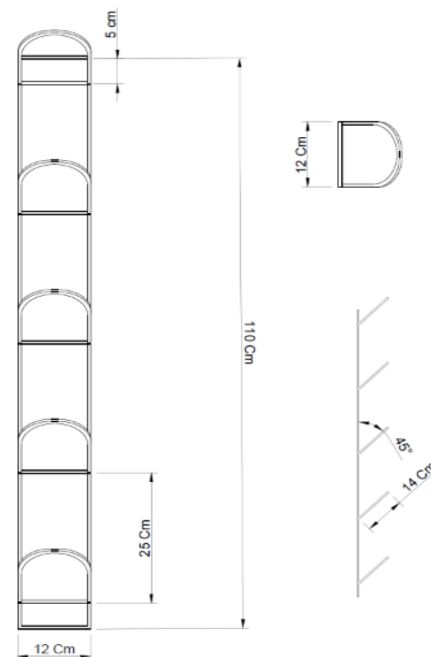
Gambar 2. Gambar Rangka Gantungan Helm Model 1
