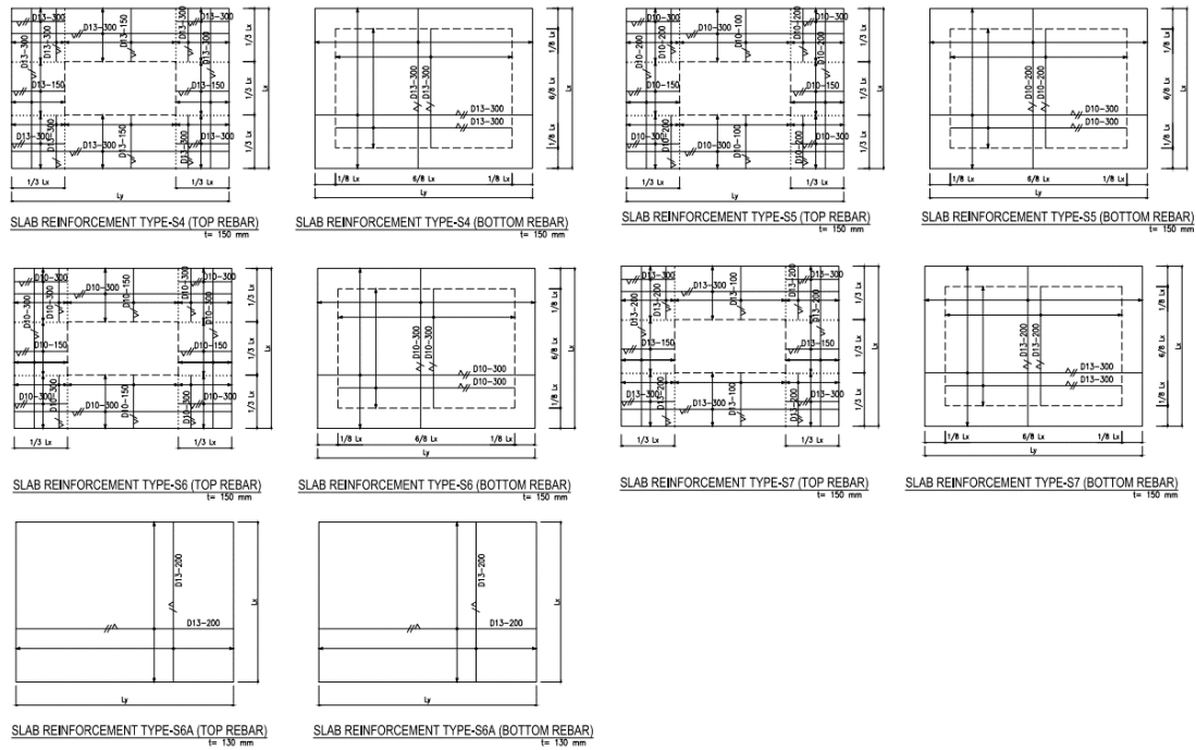
Gambar 2. Gambar kerja pelat konvensional
