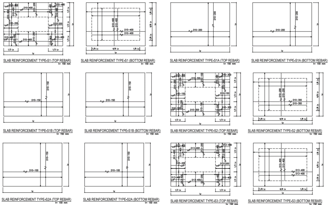
Gambar 1. Gambar kerja pelat bondek
