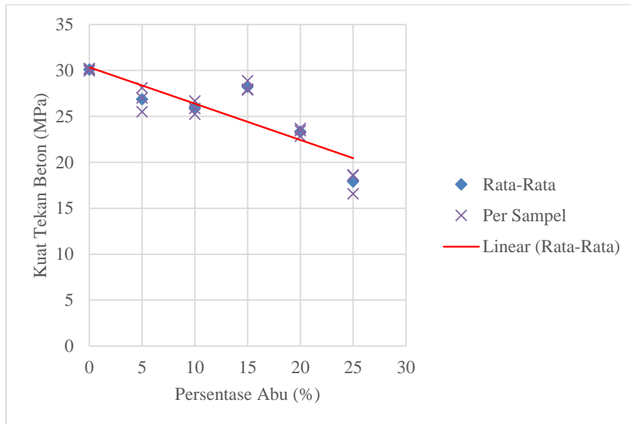
Gambar 2. Grafik hubungan antara kuat tekan beton dengan persentase abu cangkang sawit
