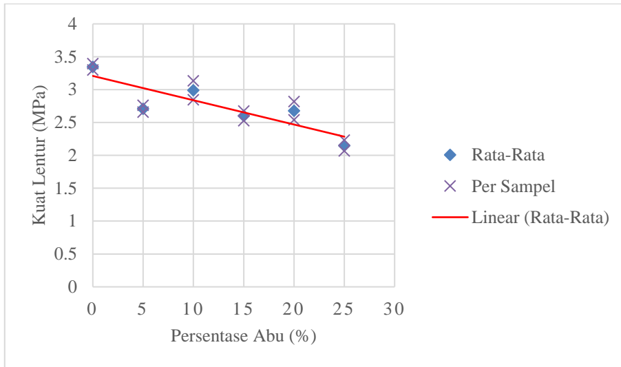
Gambar 5. Grafik hubungan antara kuat lentur beton dengan persentase abu cangkang sawit
