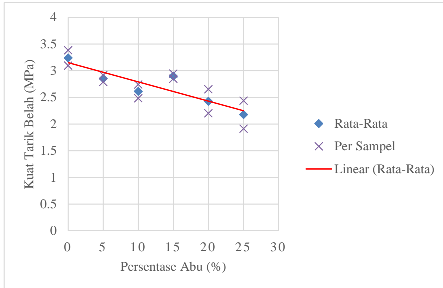
Gambar 3. Grafik hubungan antara kuat tarik belah beton dengan persentase abu cangkang sawit
