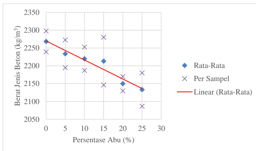
Gambar 1. Grafik hubungan antara berat jenis beton dengan persentase abu cangkang sawit
