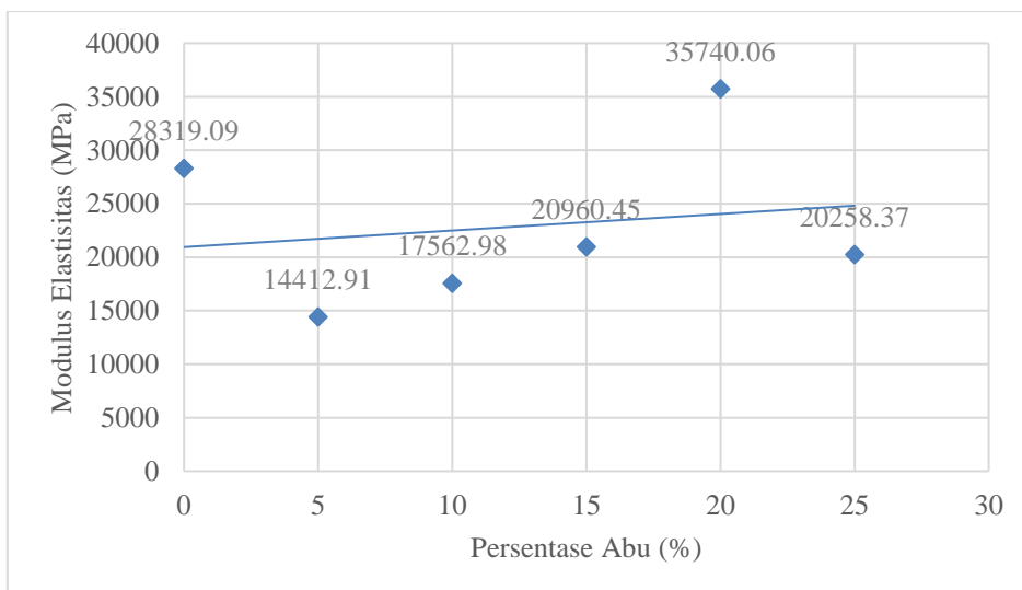
Gambar 6. Grafik hubungan antara modulus elastisitas beton dengan persentase abu
