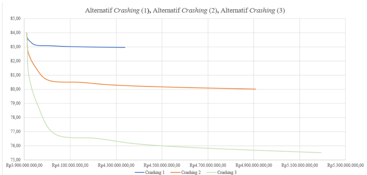
Gambar 7. Hubungan waktu dengan biaya pada 3 alternatif penambahan jam lembur
