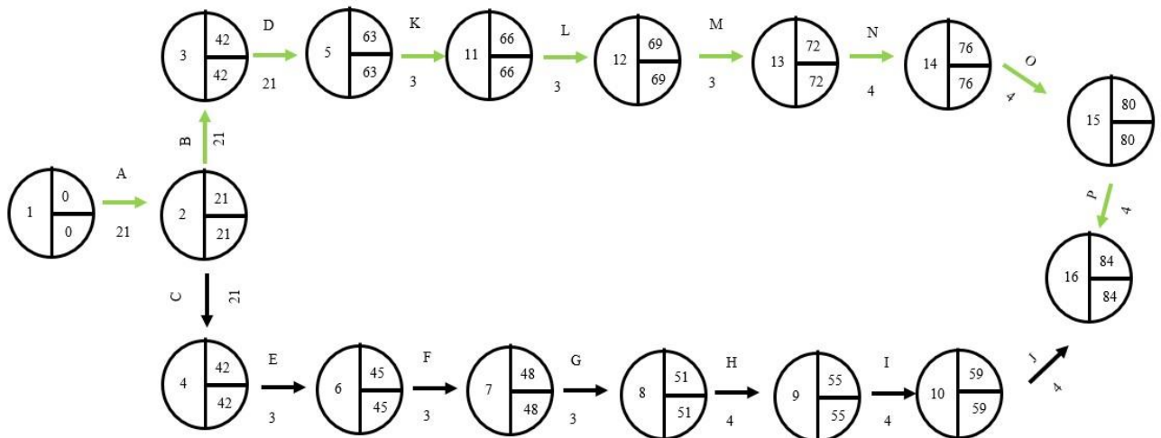
Gambar 3. Diagram critical path method untuk durasi normal
