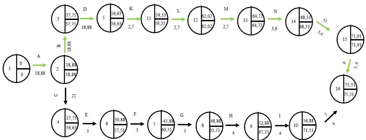
Gambar 6. Penentuan crashing alternatif 3. Hubungan waktu dengan biaya
