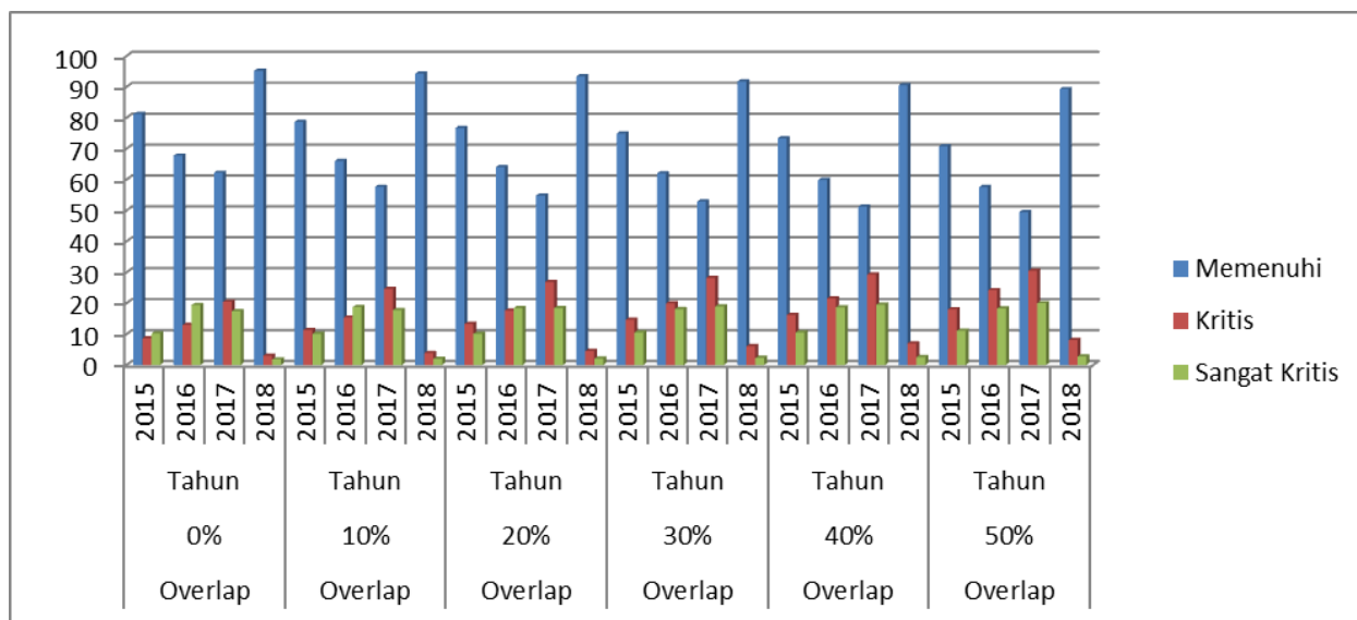
Gambar 5. Kondisi Tingkat Kekritisan Mutu Beton Sumber: Penulis, 2019
