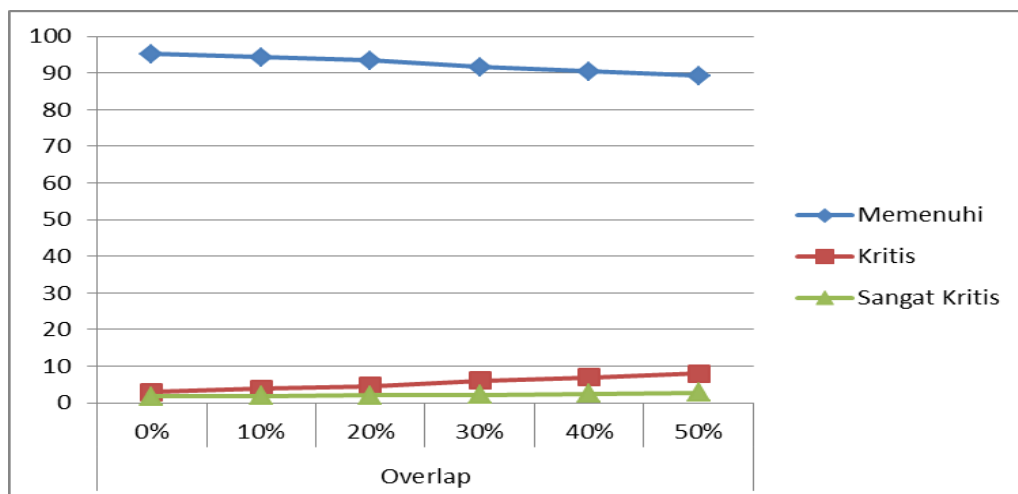
Gambar 4. Identifikasi Tingkat Kekritisan Mutu Beton Tahun 2018 Sumber: Penulis, 2019
