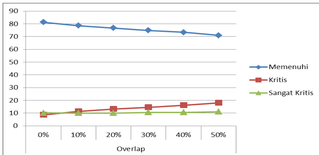
Gambar 1. Identifikasi Tingkat Kekritisan Mutu Beton Tahun 2015 Sumber: Penulis, 2019
