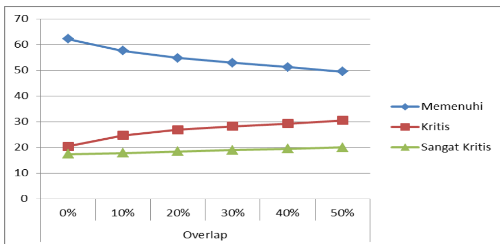
Gambar 3. Identifikasi Tingkat Kekritisan Mutu Beton Tahun 2017 Sumber: Penulis, 2019
