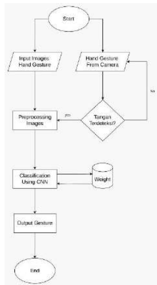
Gambar 1 Flowchart Pelatihan dan Pengujian
