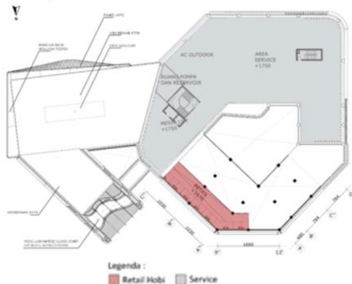
Gambar 20. Denah Lantai Service Re-desain Pasar Santa Sumber: Dokumen Pribadi, 2022
