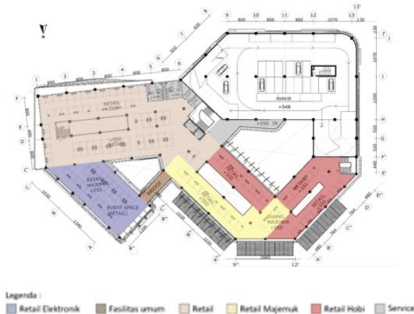
Gambar 17. Denah Lantai 2 Re-desain Pasar Santa
