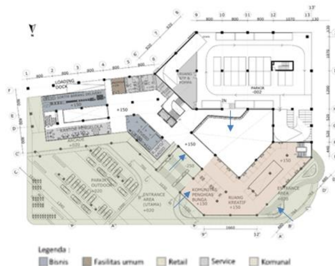
Gambar 16. Denah Lantai 1 Re-desain Pasar Santa
