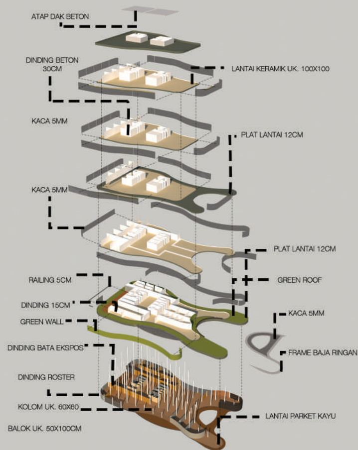
EXPLODED STRUKTUR
