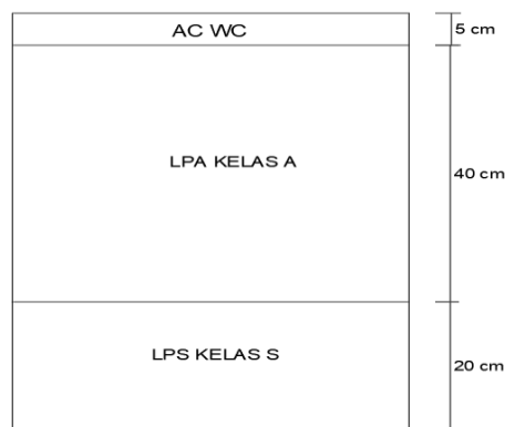
Gambar 3. Desain Tebal Perkerasan Bagian 3B
