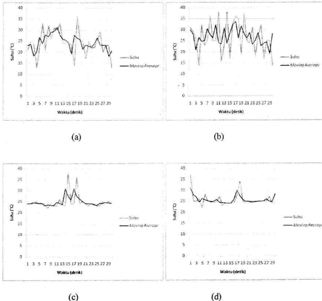
Gambar 9. Grafik Pengujian Suhu (a) Pertama, (b) Kedua, (c) Ketiga dan (d) Keempat Terhadap Waktu Selama 30 Detik
