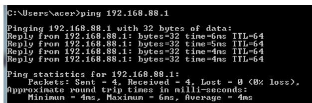
Gambar. 7 Hasil Ping Komputer 2 ke Router MikroTik
