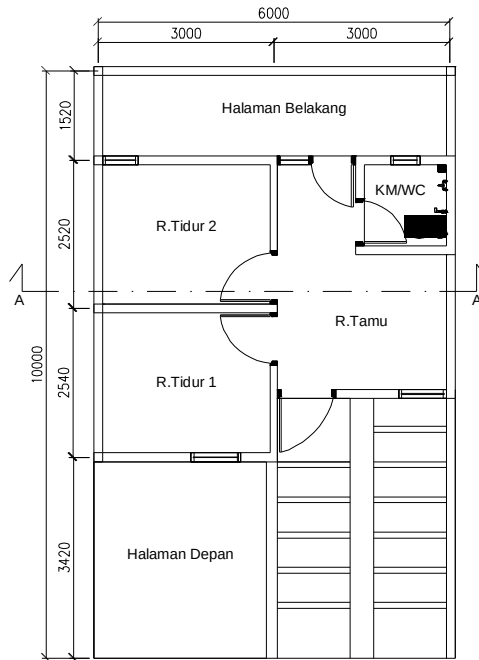
Gambar. 3 Denah Studi Kasus (Scale to Fit) Sumber: Survei, Agustus 2018
