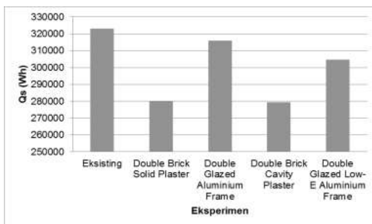
Gambar.6 Perolehan Solar Heat Gain (Qs) dalam 1 Tahun
