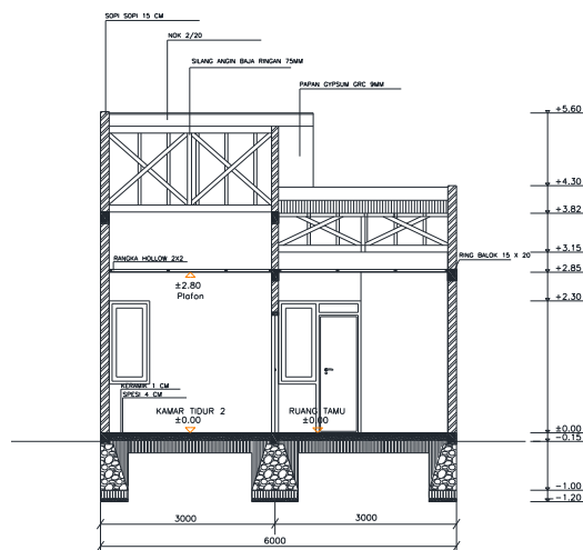
Gambar.4 Potongan A-A Studi Kasus (Scale to Fit) Sumber: Survei, Agustus 2018
