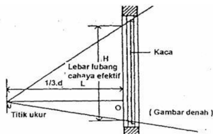
Gambar 1. Tinggi dan lebar cahaya efektif
