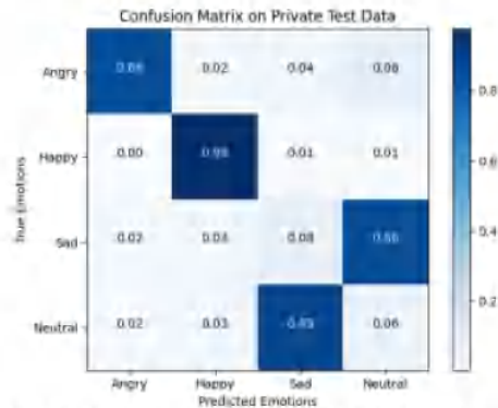
Gambar 9 Confusion Matrix pada Model VGG-16 (200 epoch)
