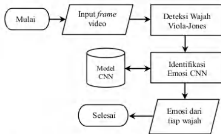
Gambar 1 Skema Perancangan Sistem Identifikasi Emosi
