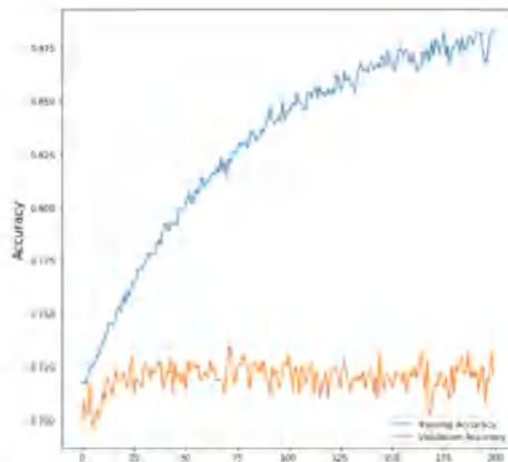
Gambar 7 Grafik Accuracy pada Model VGG-16 (200 epoch)
