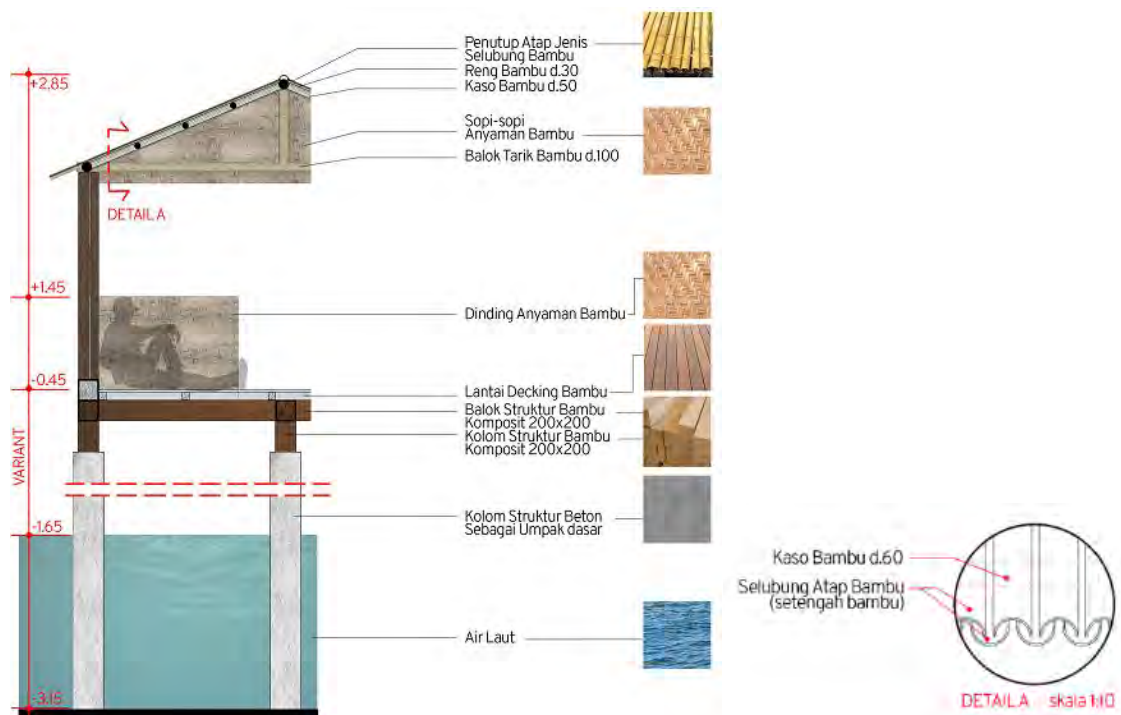
Gambar 6. Potongan Rumah Panggung Sumber: Olahan Pribadi, 2020
