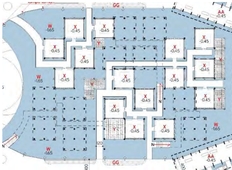
Gambar 5. Denah Rumah Panggung Sumber: Olahan Pribadi, 2020
