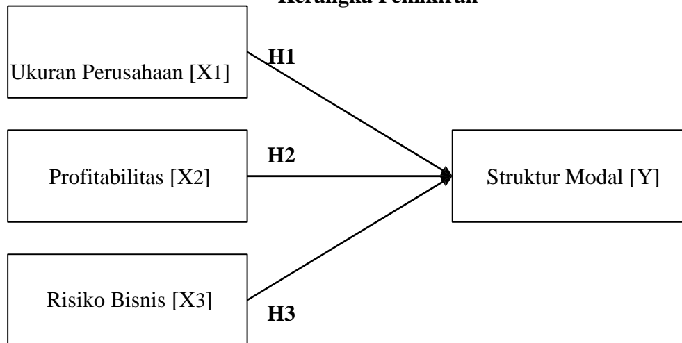
Gambar 1 Kerangka Pemikiran
