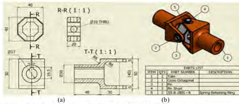
Gambar 4. (a) Pemberian dimensi pada gambar 2D dan (b) 3D
